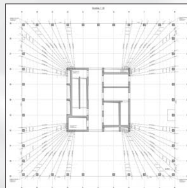
Grundriss 7. bis 16. OG
