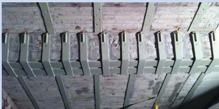
Unterzugverstärkung
